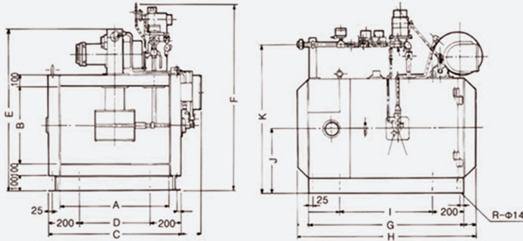
제품치수 (Dimensions)
